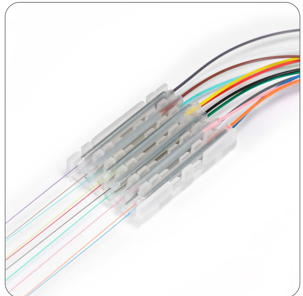
Mini Fiber Splice Holder Loaded
