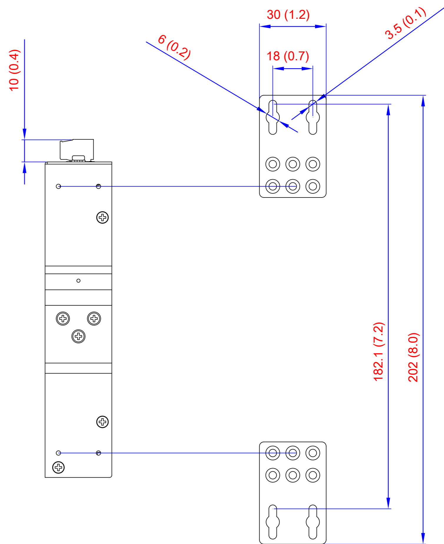
DIN Rail
